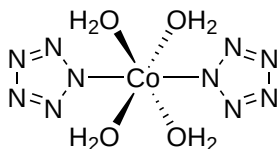
图 6: \text{Co}(\text{N}_5)_2(\text{H}_2\text{O})_4 的结构
